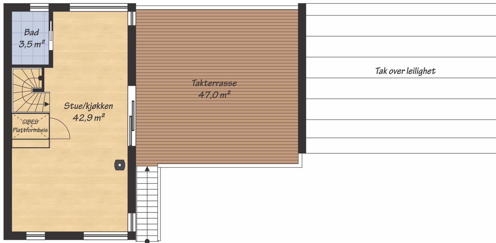
Bjørndalen Terrassen 1 - 2. Etasje uten møblering
